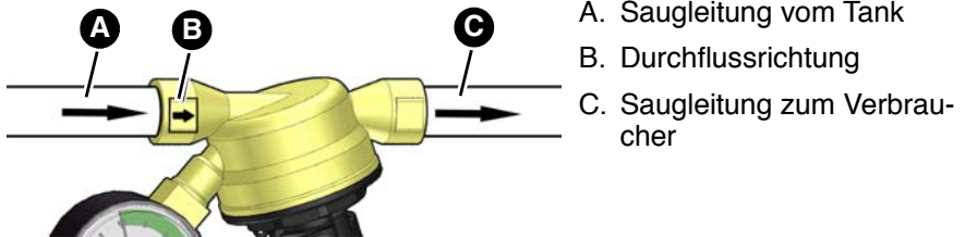
Abbildung 4: Einbau
