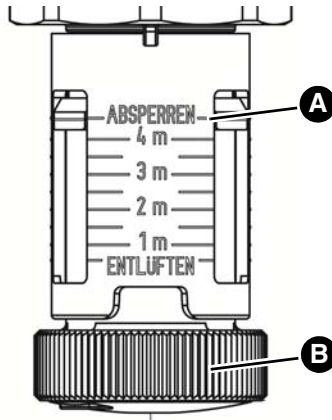
Abbildung 8: Einstellung „Absperren“
