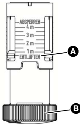
Abbildung 5: Einstellung „Entlüften“
