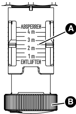
Figure 6: Hauteur de protection = différence de hauteur entre le niveau maximum dans le réservoir et le point le plus bas de la conduite d'alimentation
